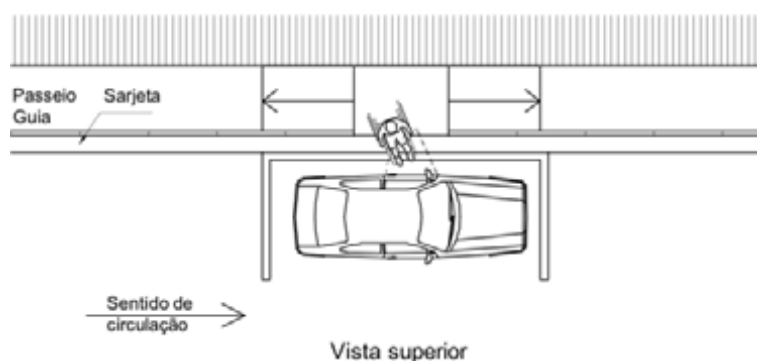
Figura 112 — Vagas para estacionamento junto a um passeio rebaixado
